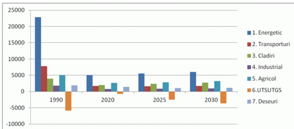
Figura 3.1. Emisiile sectoriale de gaze cu efect de seră direct în Republica Moldova în cadrul scenariului cu măsuri (necon condiționat) pentru perioada pînă în anul 2030,
