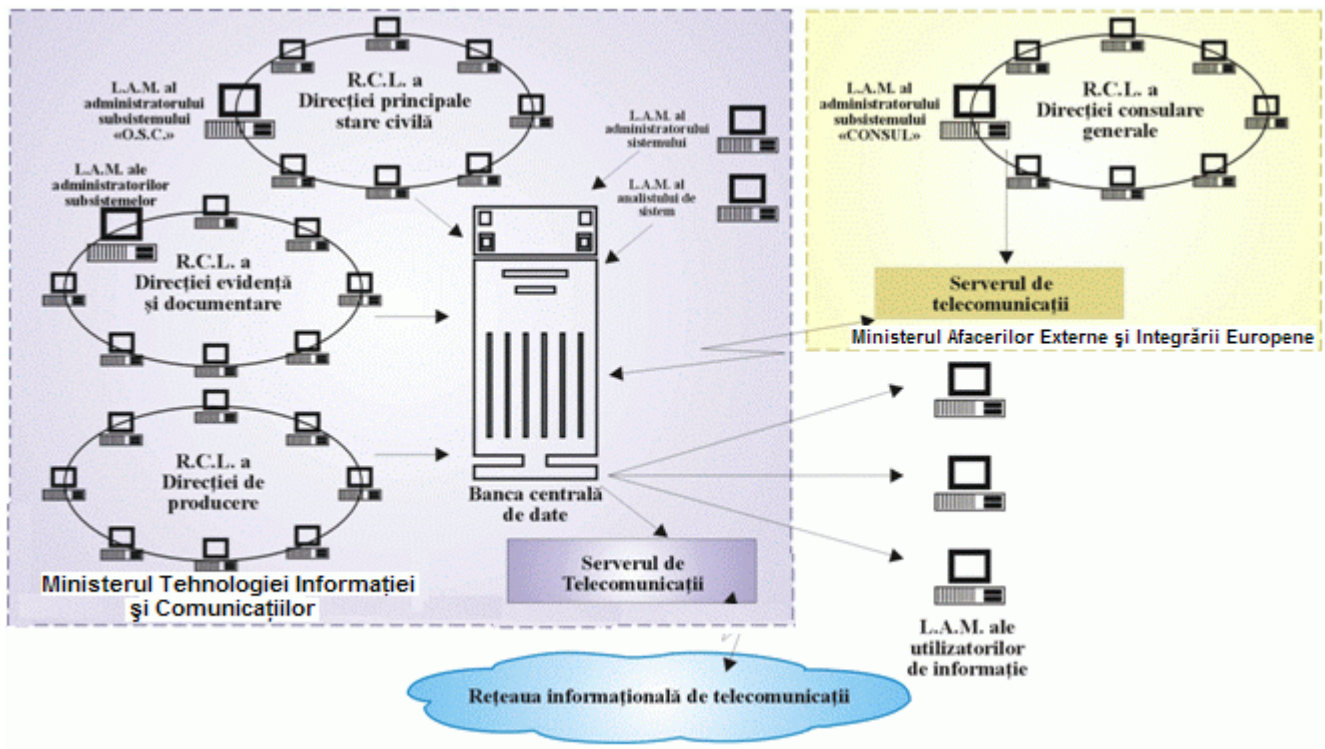
Des.18. Complexul informațional de telecomunicații de nivel central.
